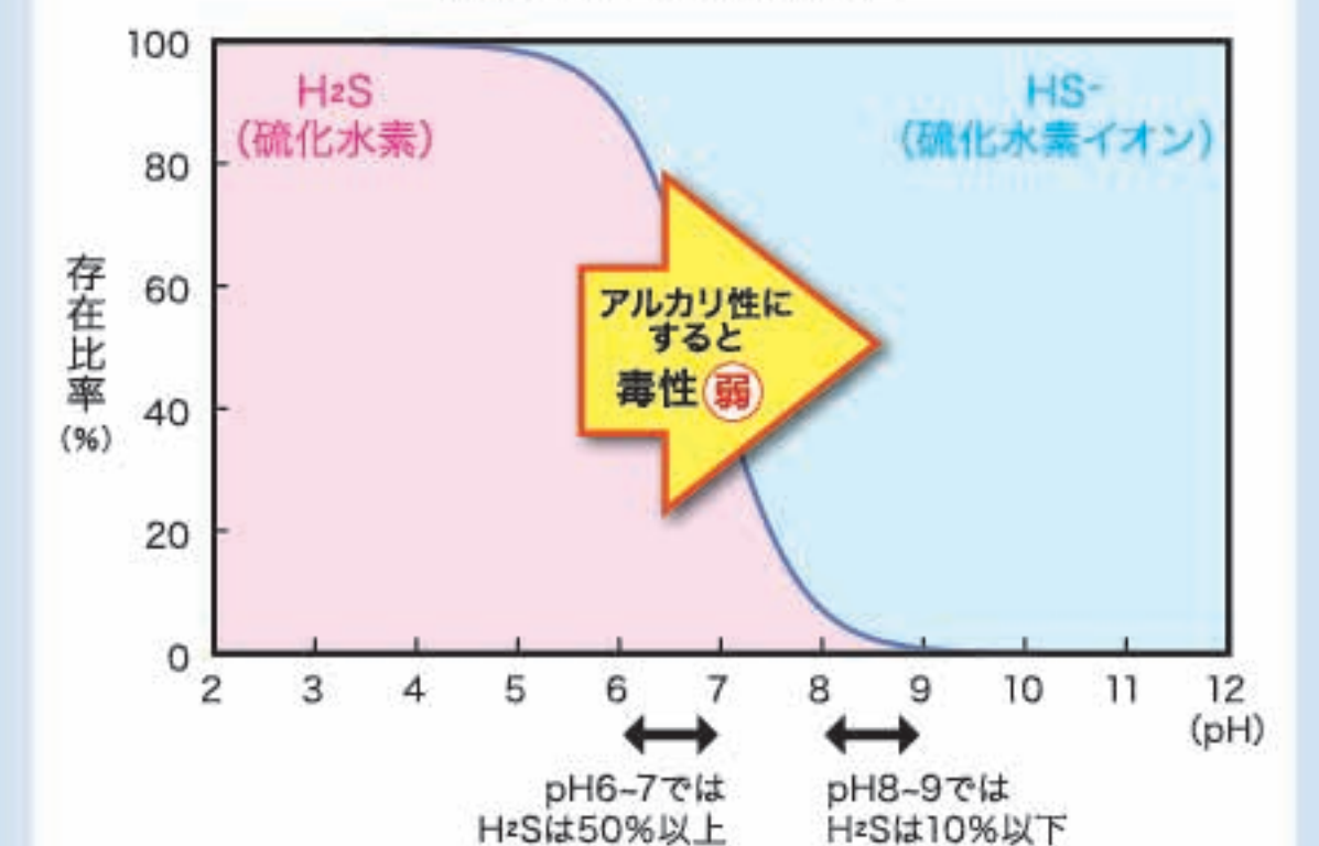
【硫化水素の存在比】
